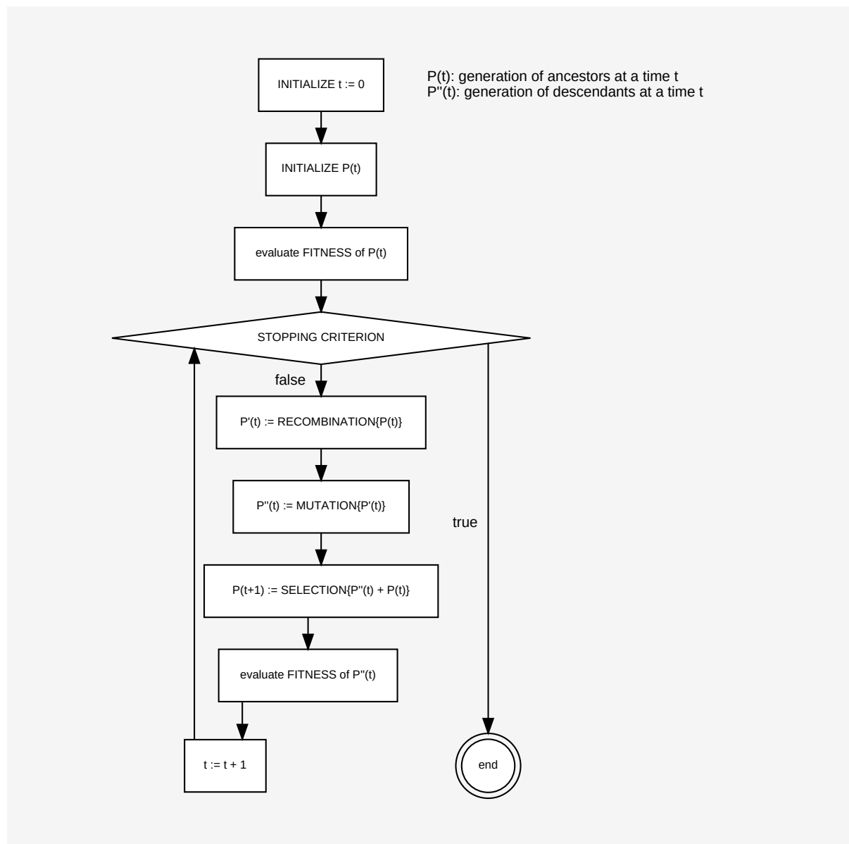
図60.1 遺伝的アルゴリズムの構造
